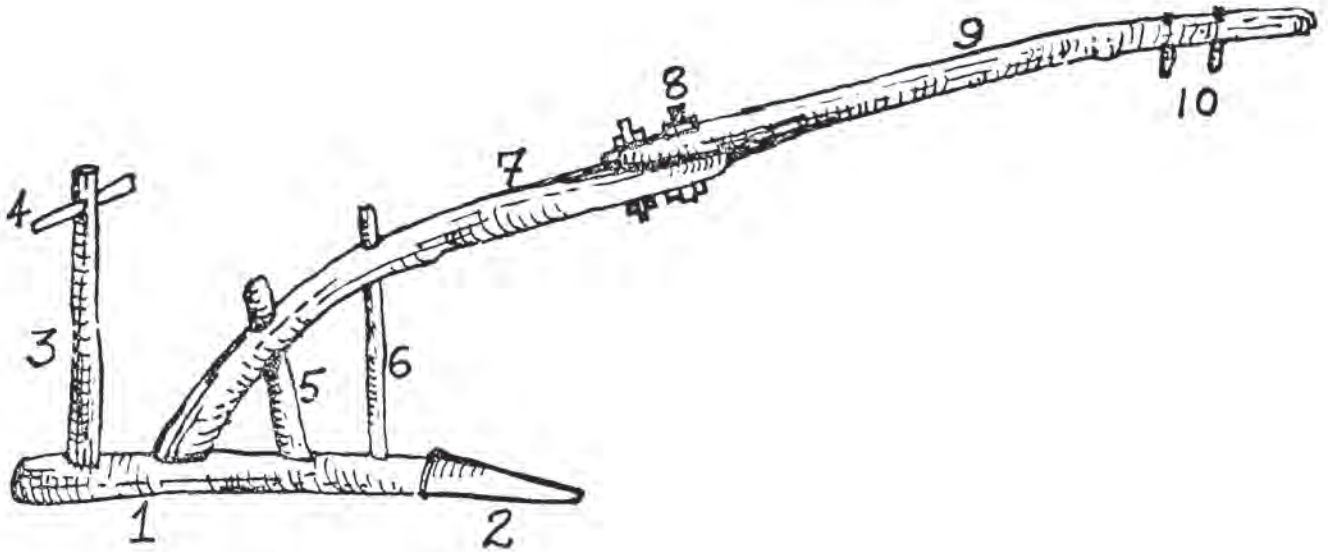
1. Ποδάρι. 2. Νίν (ύνιον). 3. Άδρωπος. 4. Σιερόσυν (λαβή). 5. Φτερό. 6. Σπάθη. 7. Βούλλα. 8. Βίδα. 9. Άμμάτισμα. 10. Κορονί.
